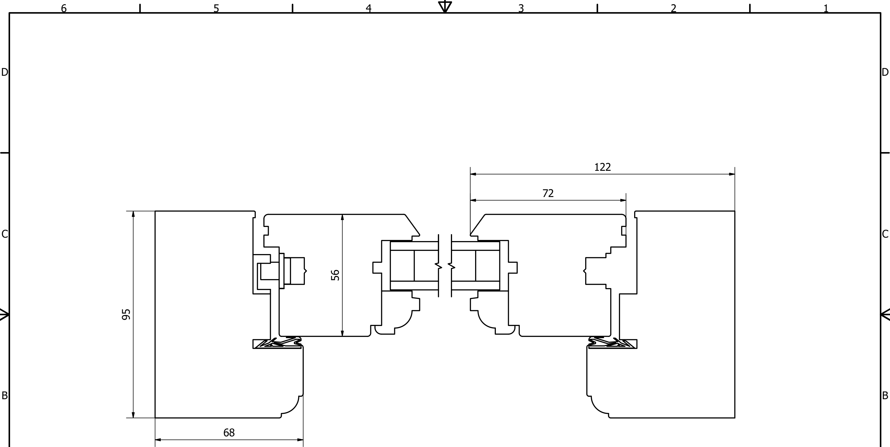
Okno casement GU - przekrój poziomy
