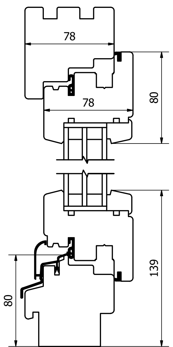
Okno ENERGO 78 profil standard - przekrój pionowy
