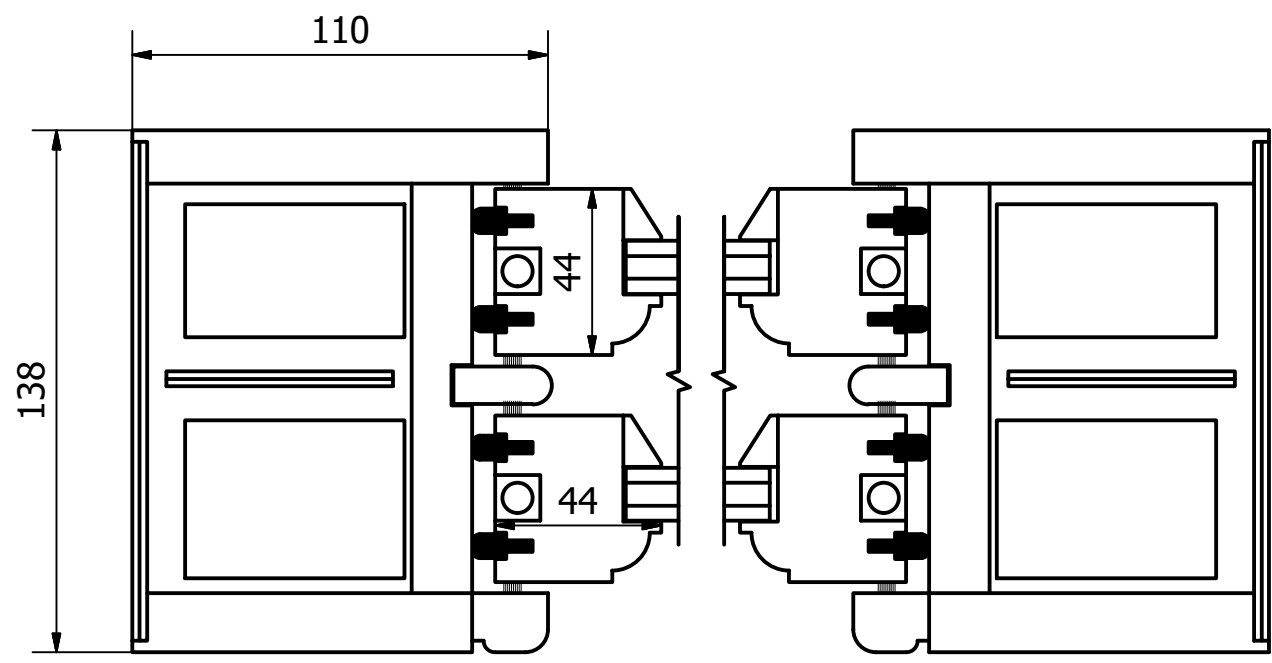
Sash 138 ciężarki - przekrój poziomy
