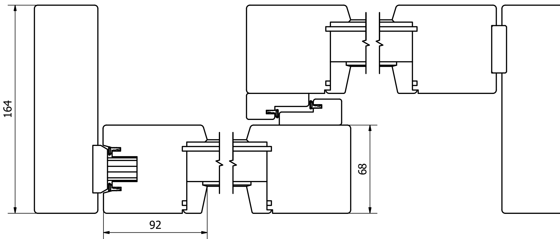
Balkon podnosząco-przesuwany HS Portal schemat A - przekrój poziomy
